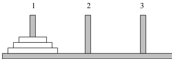
La Torre di Hanoi con n = 3 dischi.
